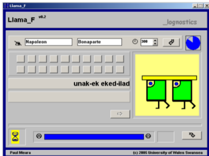
Figure 4: LLAMA_F interface
